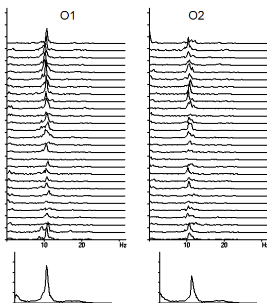
Рисунок 8 - Усредненные спектры мощности. Сверху – последовательность спектров, вычисленных для отдельных эпох длительностью 4 с у одного из испытуемых. Снизу – усредненные по эпохам спектры мощности
